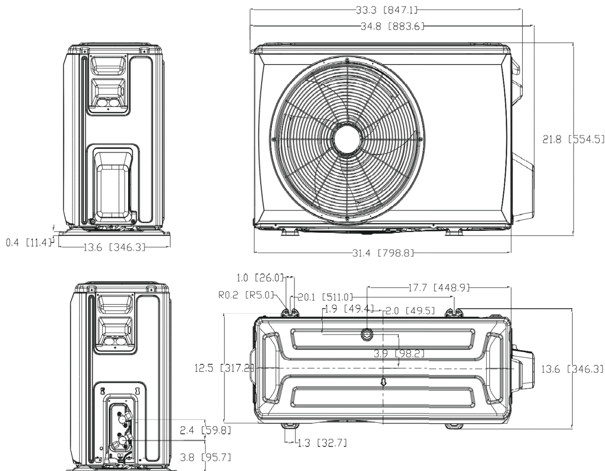
Fig. 2 – Size 18K
