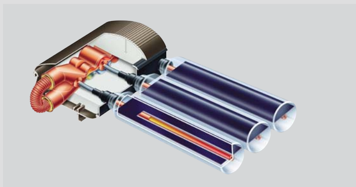
Vitosol 300-T
